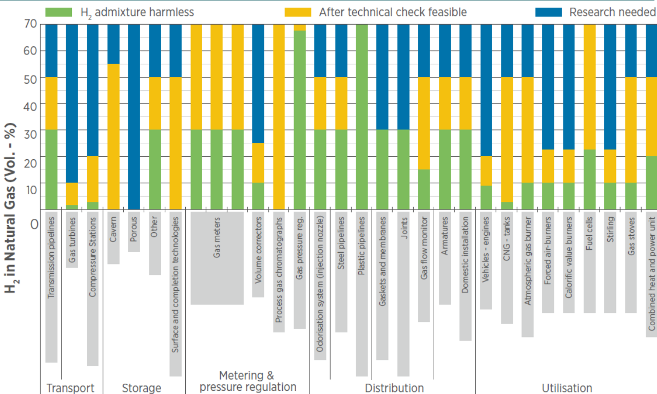
FIGURA 34 –TOLERANCA PËR HIDROGJEN E PËRBËRËSVE TË INFRASTRUKTURËS SË GAZIT
