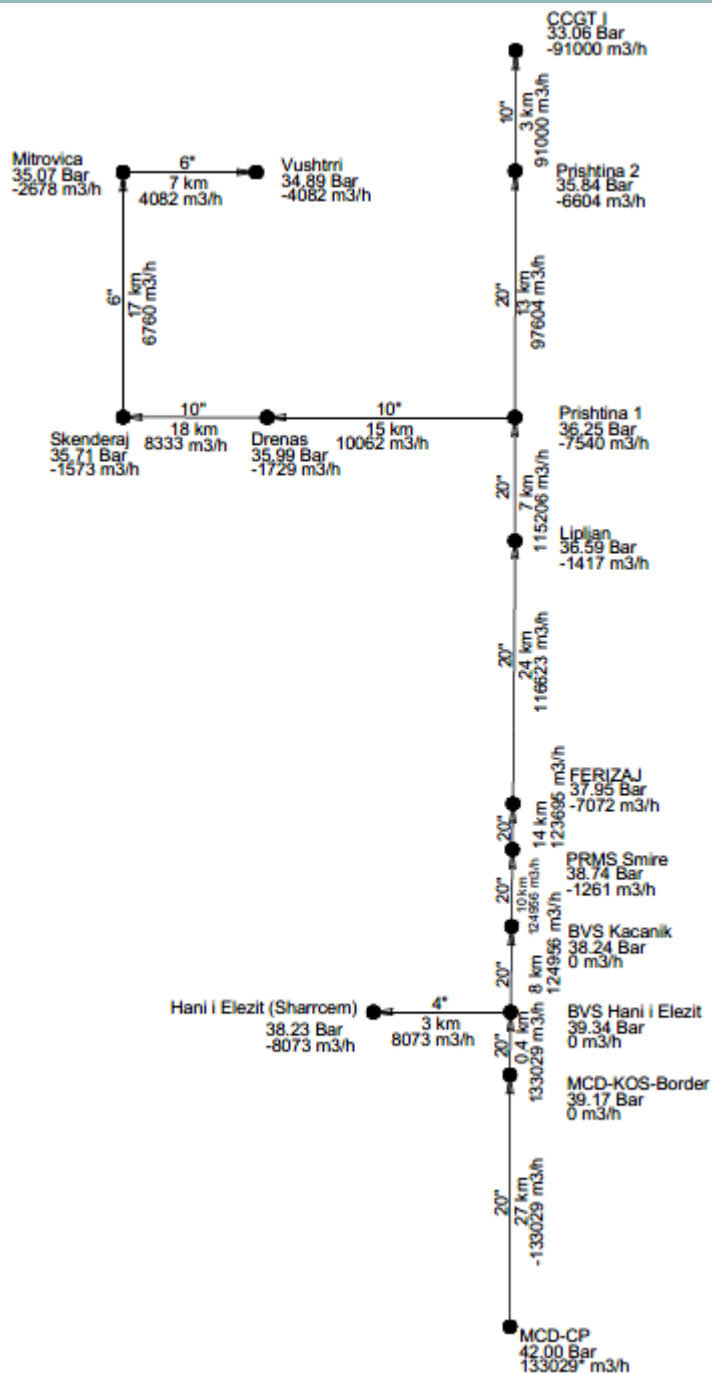
FIGURE 23 – MODELI HIDRAULIK PËR SKENARIN E GAZIFIKIMIT INDUSTRIAL
