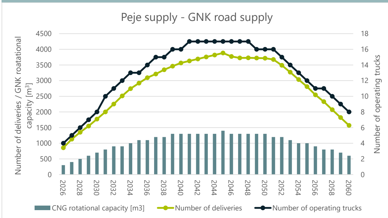
FIGURA 148 – SISTEMI I FURNIZIMIT ME GNK PËR PEJËN
