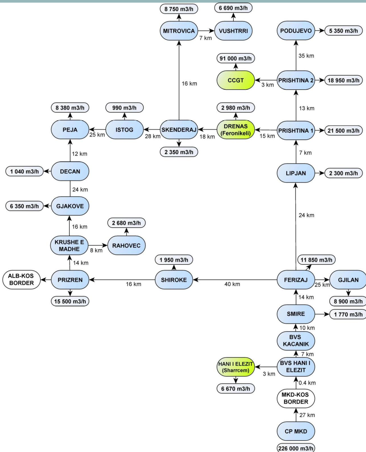
FIGURA 86 – DIAGRAMI BLOK I RRJEDHËS PËR SKENARIN E GAZIFIKIMIT NË SHKALLË TË GJERË
