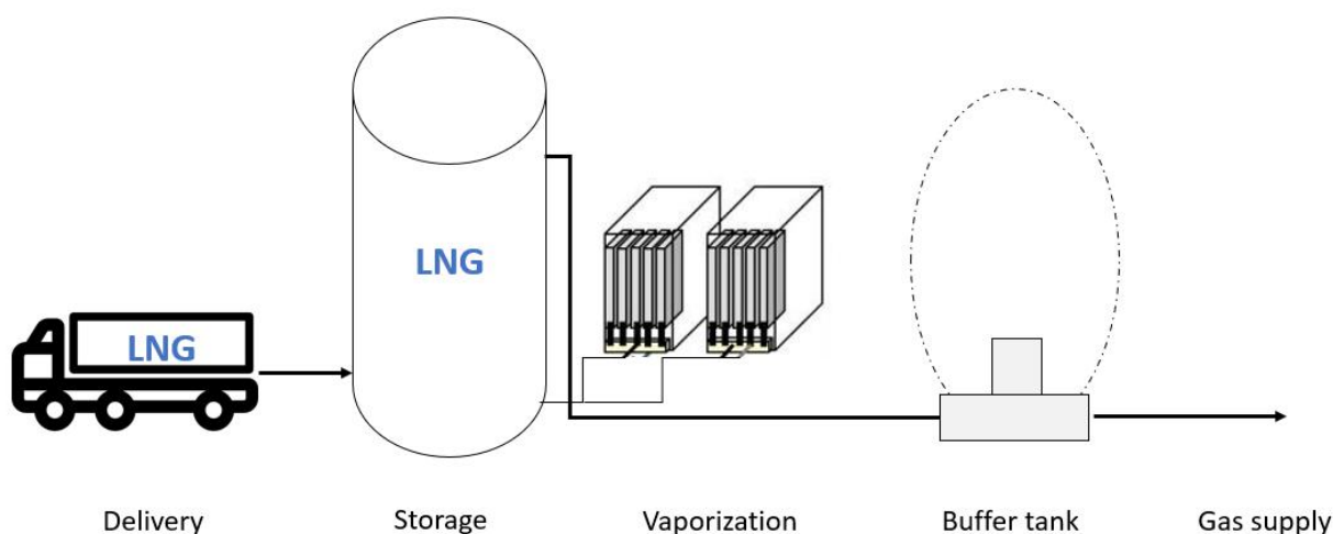
FIGURA 139 – ZINXHIRI I FURNIZIMIT ME GAZ ME GNL SI BURIM
