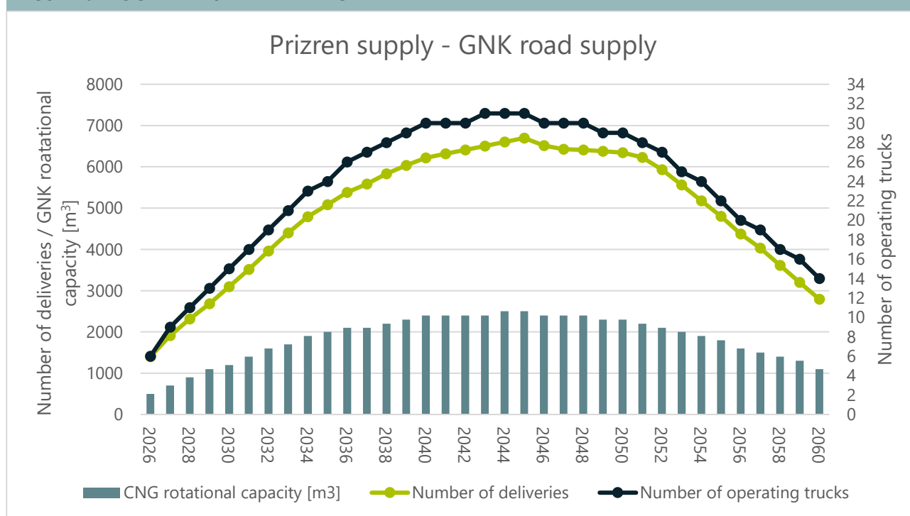
FIGURA 67 – SISTEMI I FURNIZIMIT ME GNK PËR PRIZRENIN
