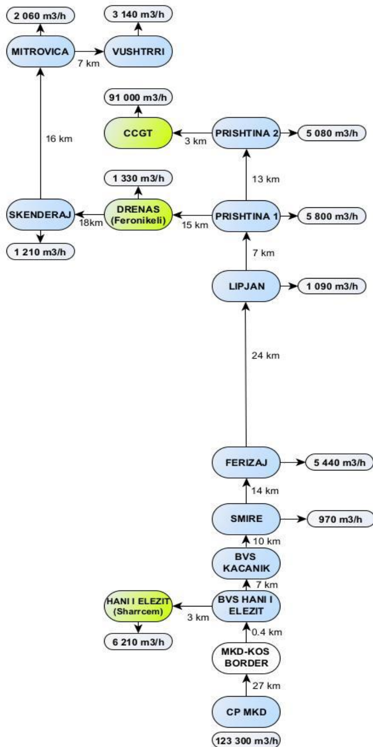
FIGURA 90 – DIAGRAMI BLOK I RRJEDHJES PËR SKENARIT E GAZIFIKIMIT TË VOGËL INDUSTRIAL
