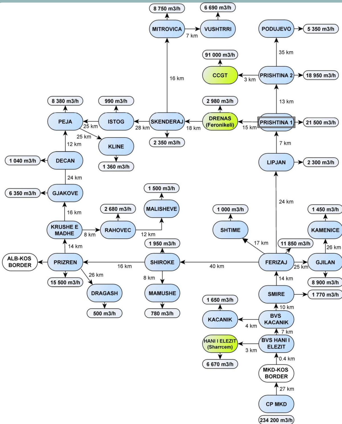
FIGURA 84 – DIAGRAMI BAZË BLOK I RRJEDHËS
