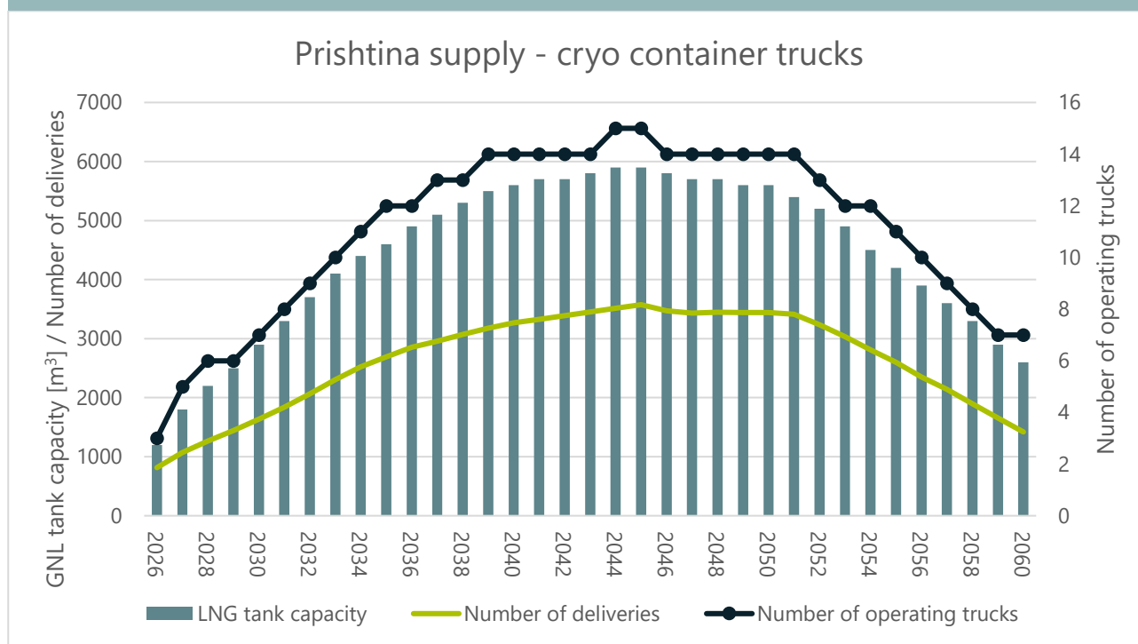
FIGURA 61 – SISTEMI I FURNIZIMIT ME GNL PËR PRISHTINËN NGA RRUGA
