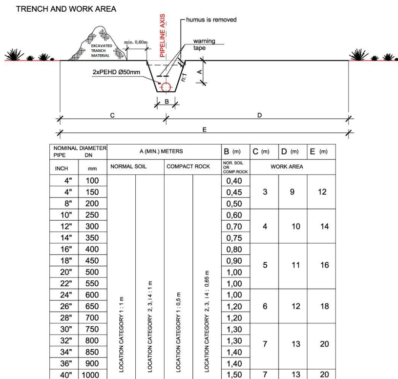
FIGURA 2816 – KANALI DHE ZONA E PUNIMEVE
