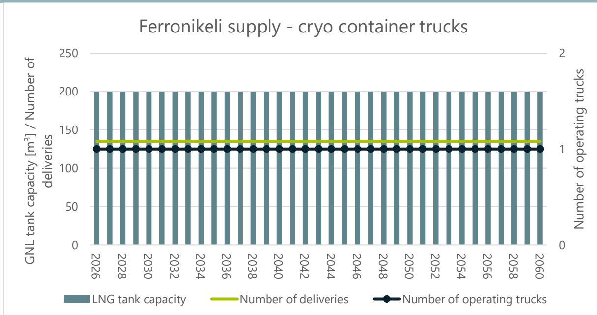
FIGURA 64 – SISTEMI I FURNIZIMIT ME GNL PËR FERRONIKELIN ME RRUGË
