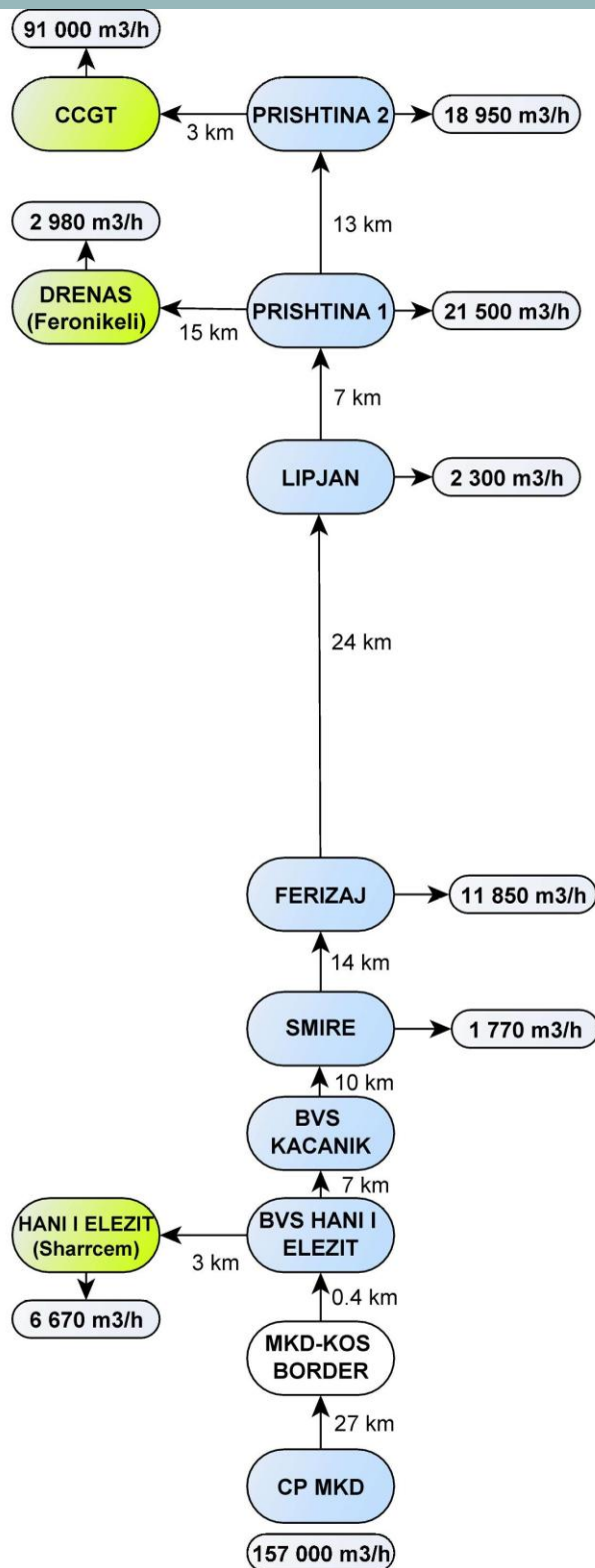
FIGURA 218 – DIAGRAMI BLOK I RRJDHËS PËR SKENARIN E GAZIFIKIMIT NË SHKALLË TË VOGËL
