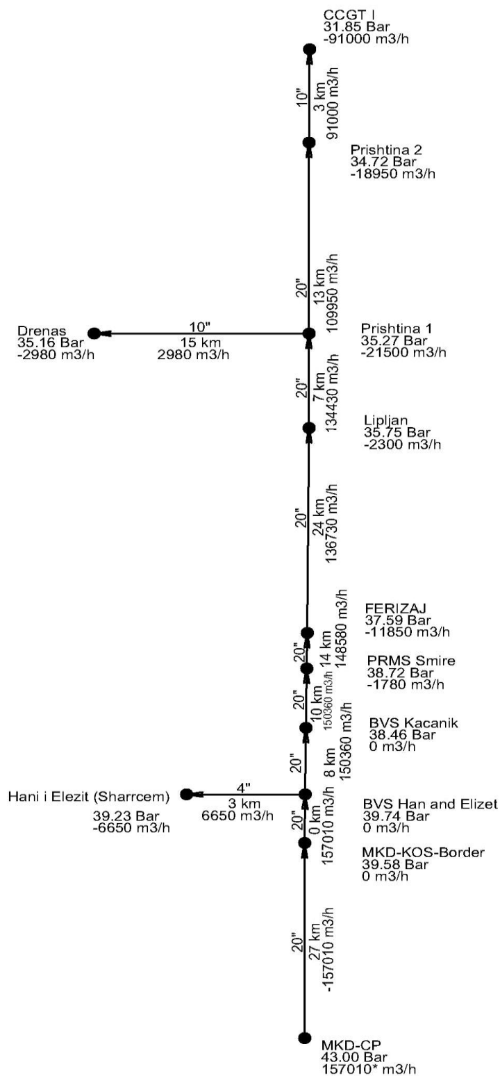
FIGURA 229 – MODELI HIDRAULIK PËR SKENARIN E GAZIFIKIMIT NË SHKALLË TË VOGËL
